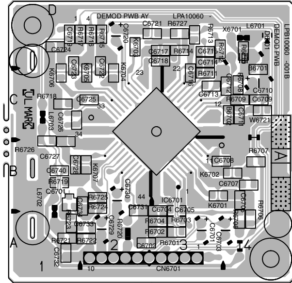
<14> DEMODULATOR LPB10060-001B
